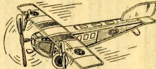
Flygmaskin № L 19, av lackerad plåt. Försedd med två urverk, det ena driver propellern och det andra hjulen, varför den går såväl på golvet som i luften om den upphängs med ett snöre. Propellern går i c:a 1½ minut med en uppdragning. Längd 35 cm., bredd med vingarna 36 cm. Pris pr st. 1:90
