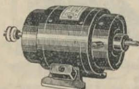
Motor N o T 401, på 1/20 hästkraft. Motors längd utom axeln c:a 12 cm., höjd c:a 10 cm. Vikt 1700 gram. Pris pr st. 24:50
