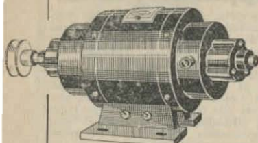
Motor N o T 403, på 1/8 hästkraft. Motors längd utom axeln c:a 21 cm., höjd c:a 12 cm. Vikt 3700 gram. Denna motor är försedd med kullager. Pris pr st. 49:75
